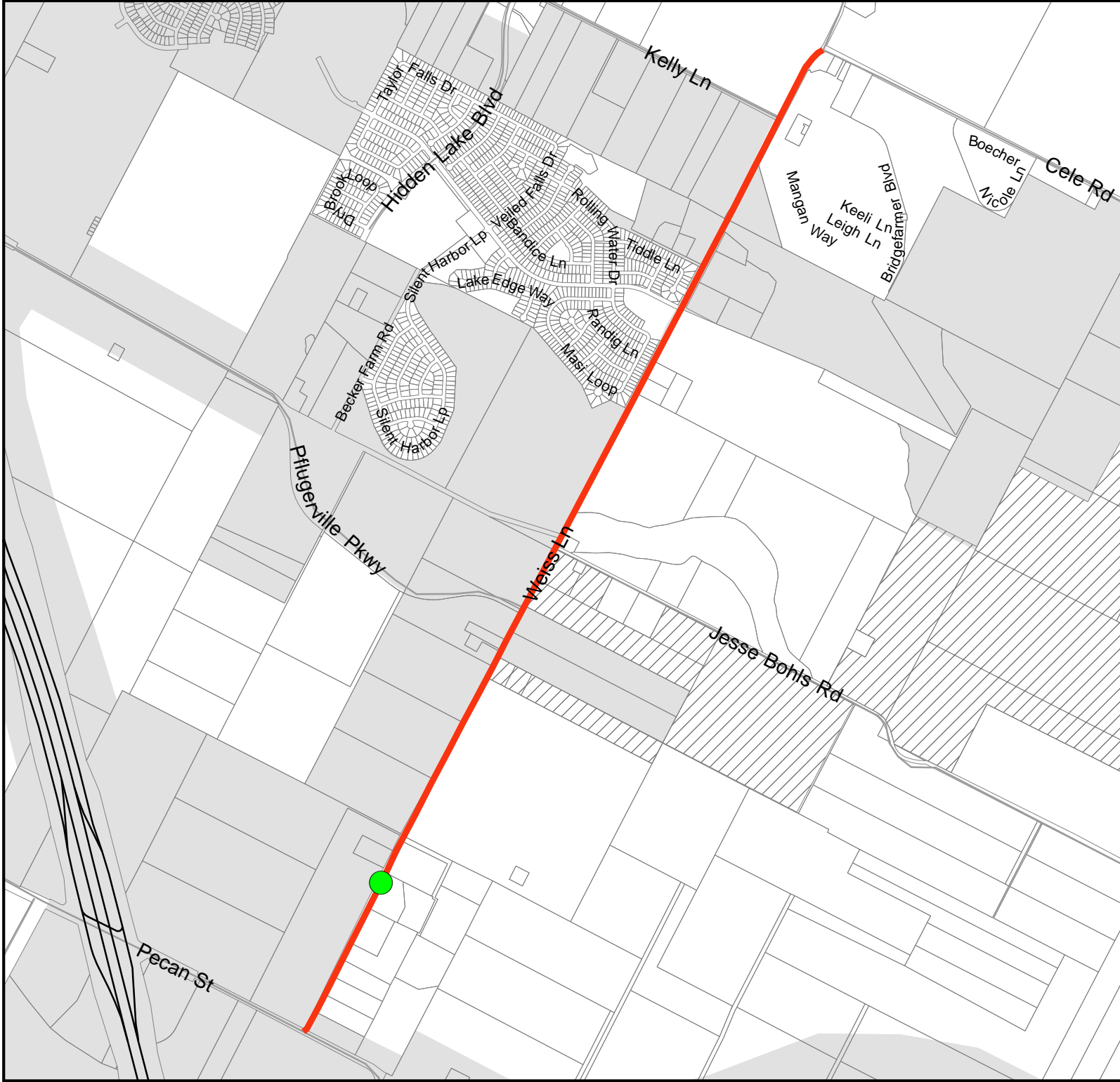
Locator Map
